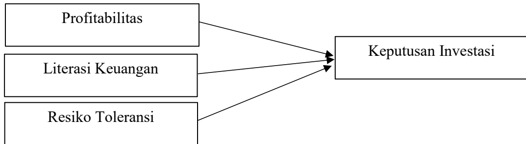
Gambar 1. Kerangka Konseptual
